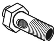
オリフィス無しタイプボルト スバル純正部品14445AA090
