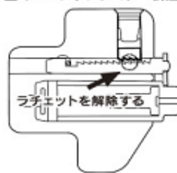
■ チェーンテンショナー構造
